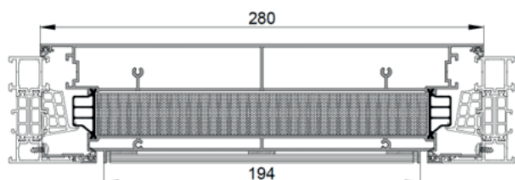
Структурная створка, L = 280 мм
