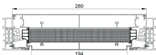
Классическая створка, L = 280 мм
