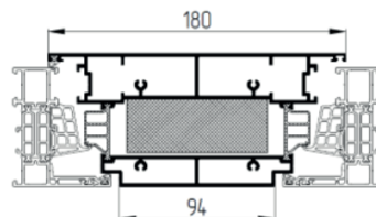
Классическая створка, L = 180 мм
